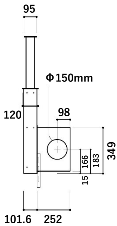
立面図(左側面)
