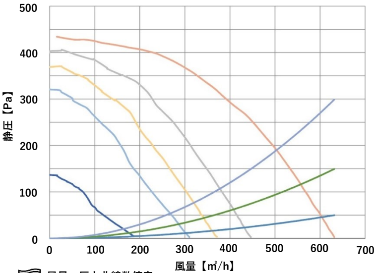
風量・圧力曲線数値表
